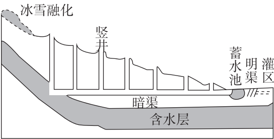
图(b) 坎儿井结构示意图
