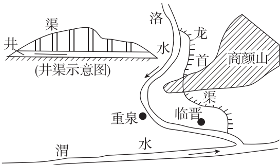
图(a) 井渠法原理示意图
